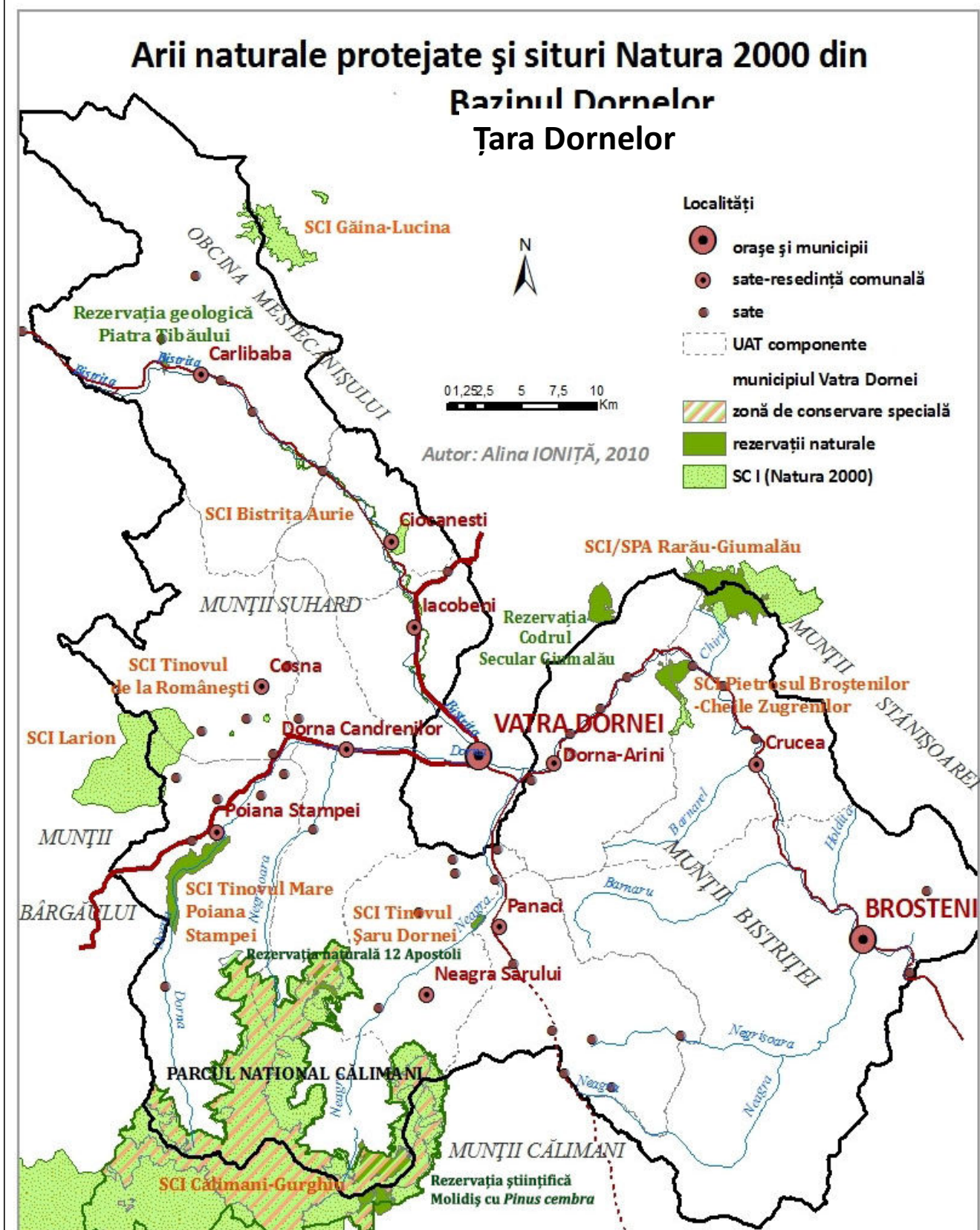
Fig. nr. 2 – Ariile naturale protejate din Bazinul Dornelor
