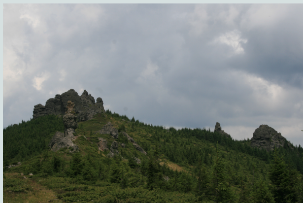
Rezervația geologică 12 Apostoli - Parcul Național Călimani
